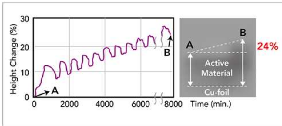
Figura 1 - Variazioni dell'altezza del materiale dell'anodo di grafite durante la carica e la scarica di una batteria agli ioni di litio (Furukawa Electric Review, No. 134 2015-1)
