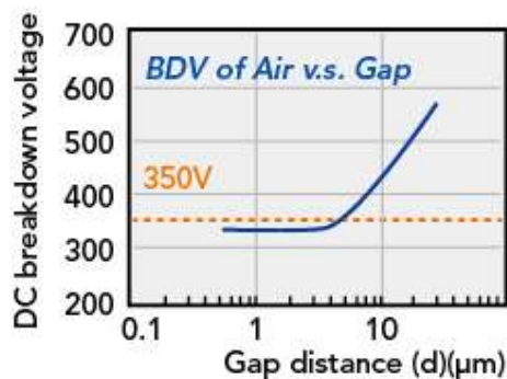
Figura 2 - Tensione di breakdown dell'aria in funzione della distanza
