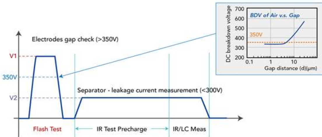
(Figure 4) Chroma 11210 + Flash Test per l'ispezione della qualità dell'isolamento delle batterie Li-ion
